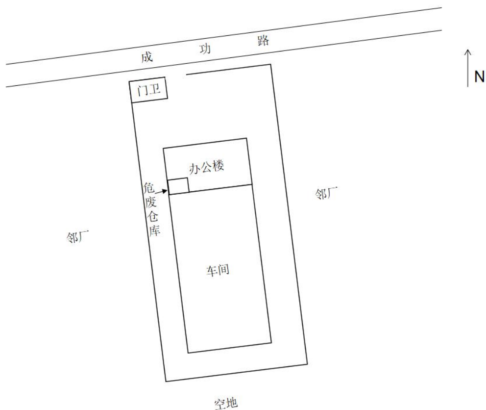
图 3-2 平面布置及危废仓库位置图
