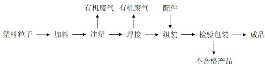
图 3-3 生产工艺流程及产污环节图
