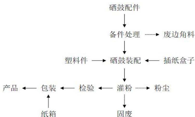
图 3-3 生产工艺流程及产污环节图
